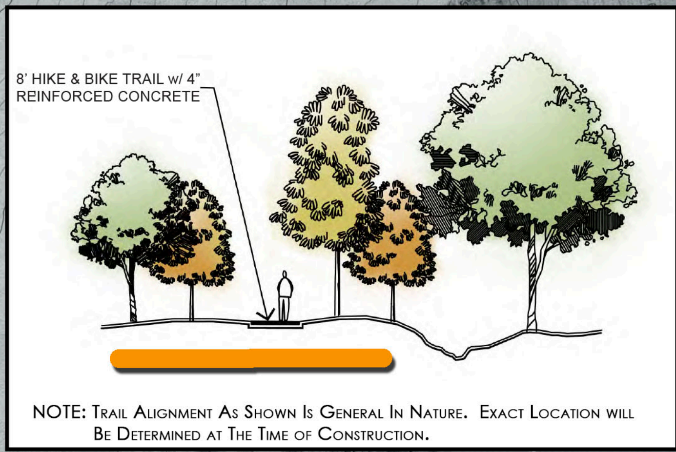
Hike & Bike Trail Section N.T.S.
